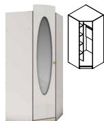
7. Шкаф угловой СБ-1868 877 x 2144 x 877 ширина бока 540
